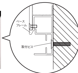
5 フレームの溝から壁面へ取り付けます。 ※壁面取付ビスは、取り付ける壁面に合わせて別途ご用意ください。
